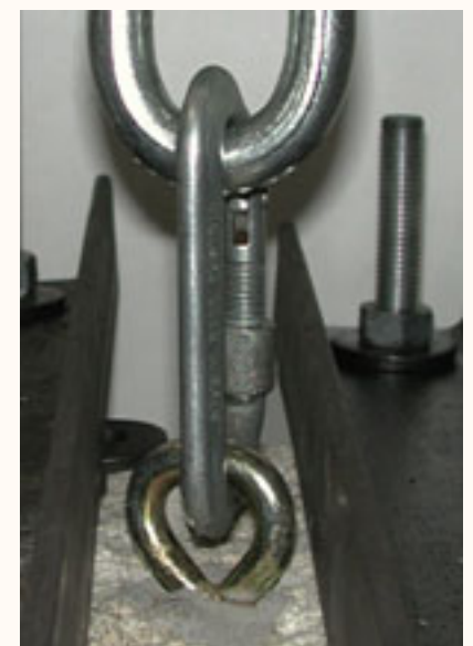
Fixation dans un bloc de granit. Exemple de traction axiale sur broche FIXE
