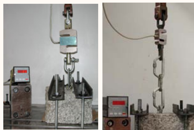
Test sur broche fixe
